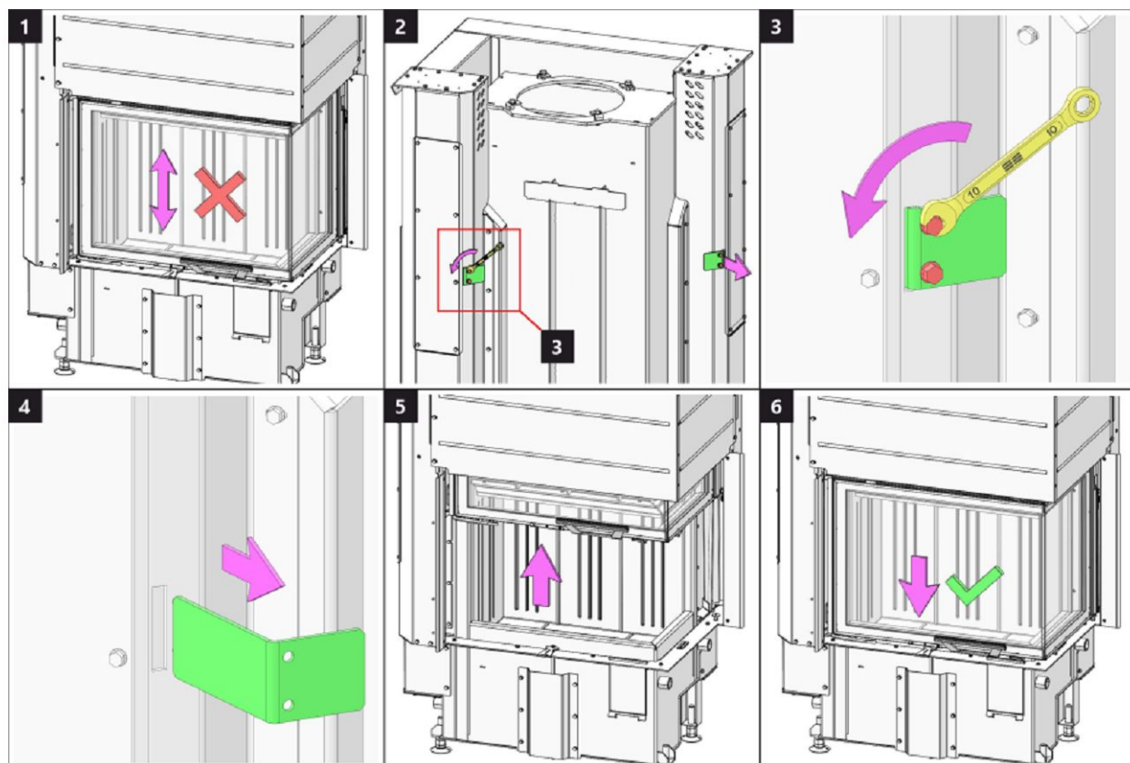
Fireplace door – Locking mechanism 1 | Feuerraumtür – Arretierung 1
